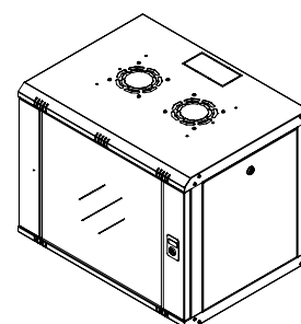
VISTA ISOMETRICA
